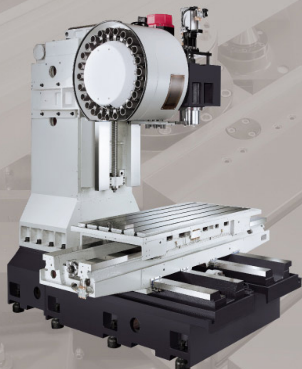
JMV-1400 機身結構
