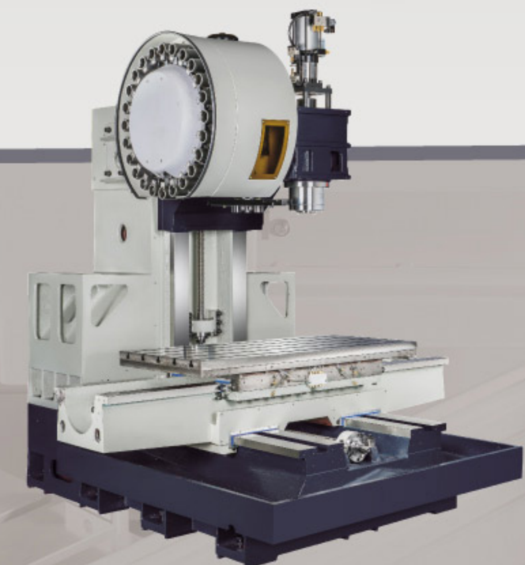
JMV-1200A 機身結構
