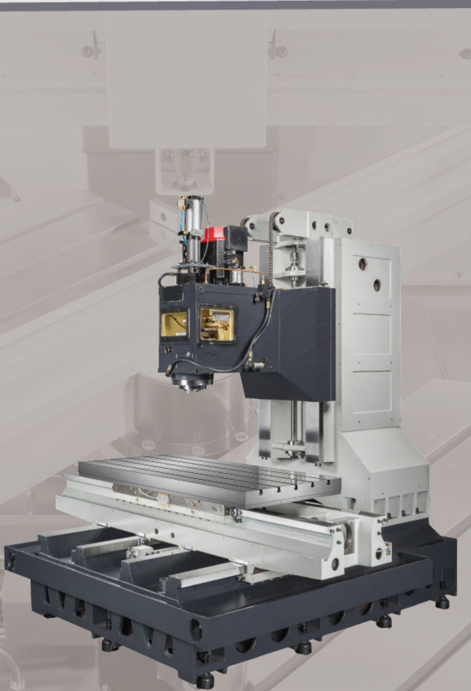
JMV-1600 / 1800 機身結構
