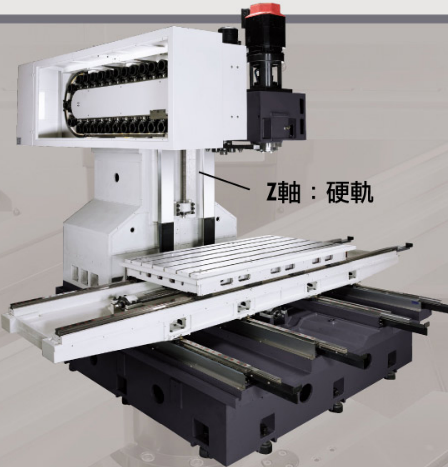
JHV-1800 / 2000 機身結構
